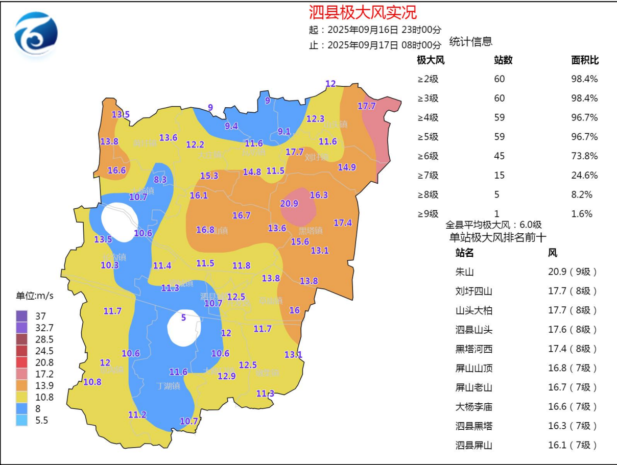
图 2 泗县 9 月 16 日 23 时至 17 日 08 时极大风实况图
