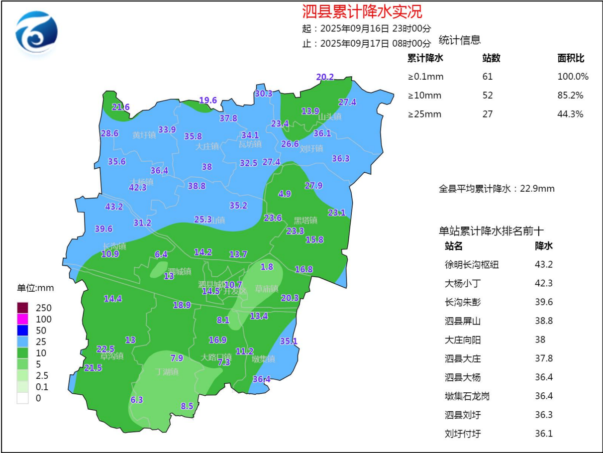
图 1 泗县 9 月 16 日 23 时至 17 日 08 时累计降雨量图
