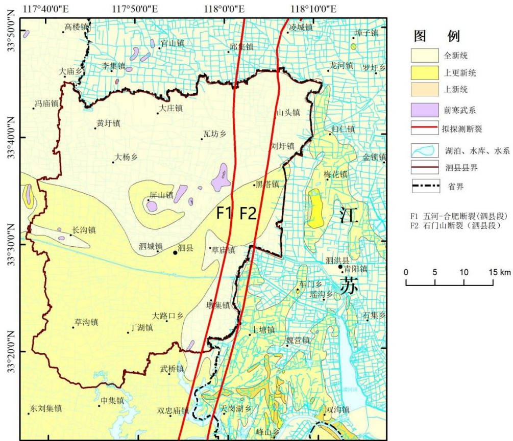
图 2.1 泗县研究区范围和主要断裂分布图
